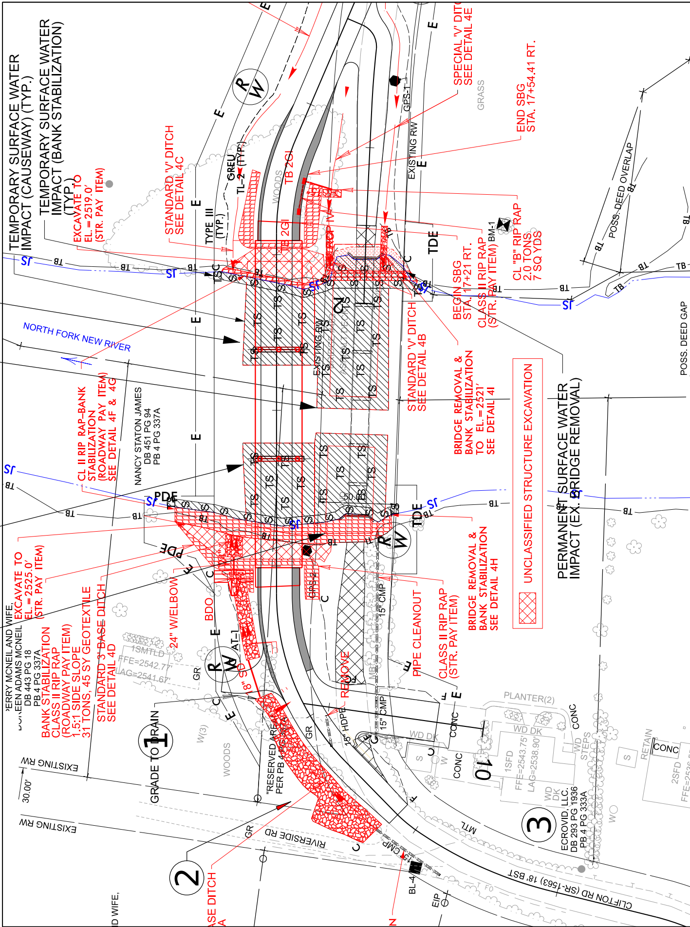
SITE 1 - ENLARGEMENT
